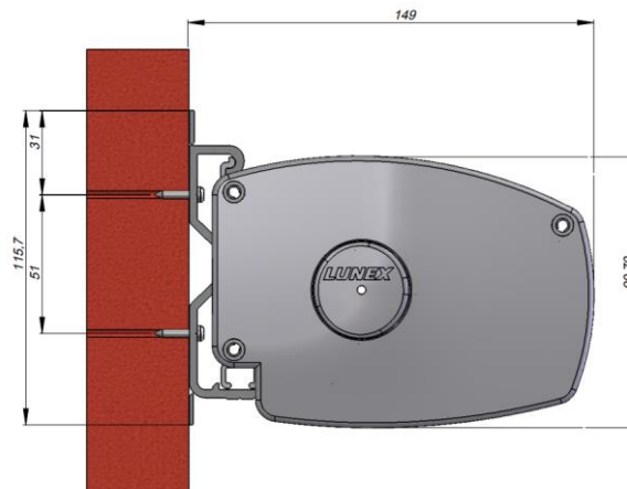
Måttskiss Optima
