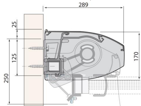
Måttskiss Takskydd
